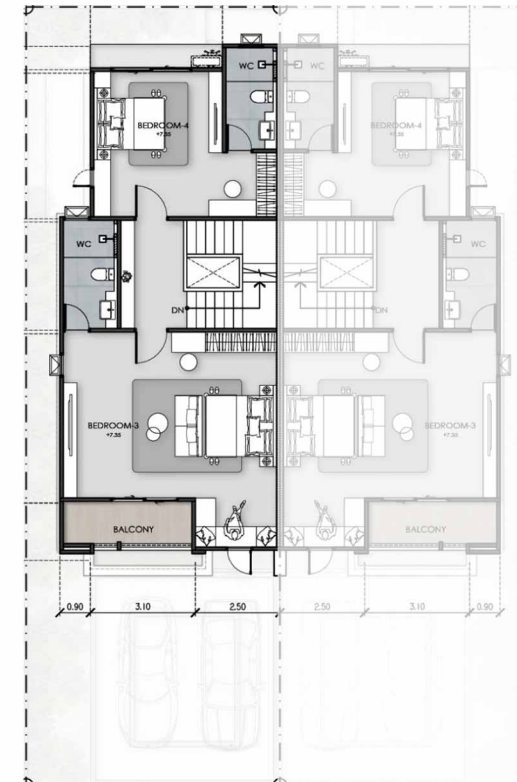
ប្លង់ជាន់ទី៣ 3 rd FLOOR PLAN
