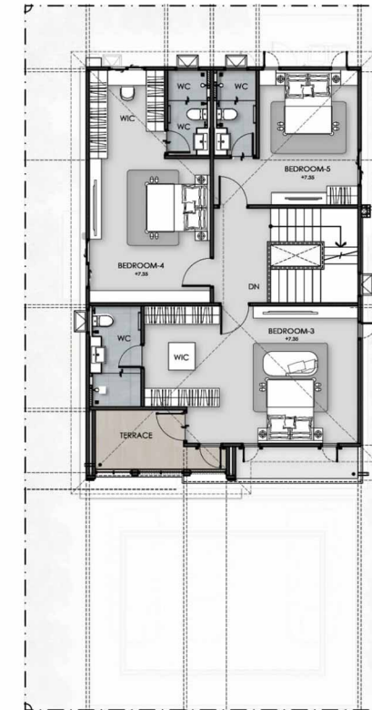
ប្លង់ជាន់ទី៣ 3rd FLOOR PLAN
