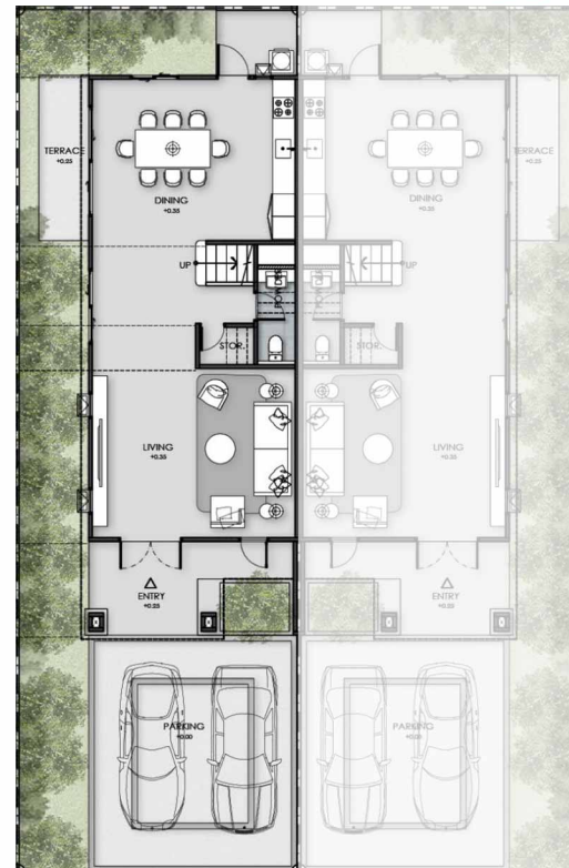
ប្លង់ជាន់ផ្ទាល់ដី 1 st FLOOR PLAN
