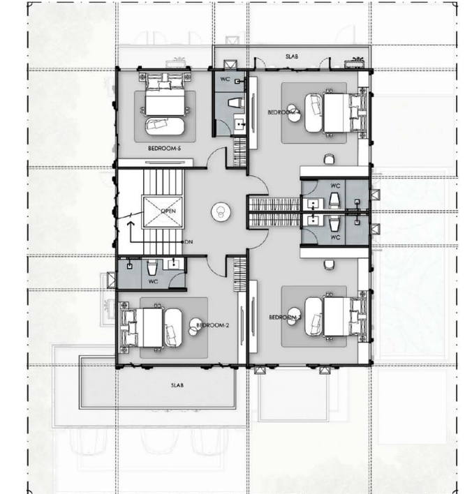
ប្លង់ជាន់ទី៣ 3rd FLOOR PLAN
