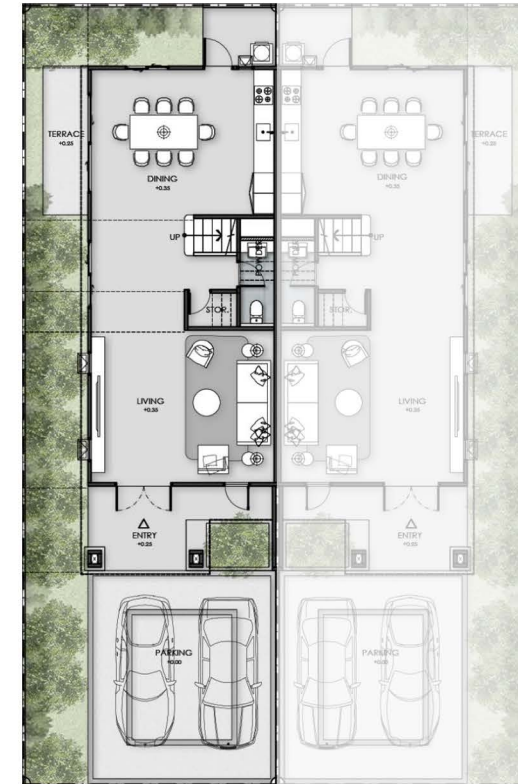
ប្លង់ជាន់ថ្នាលដី 1st FLOOR PLAN
